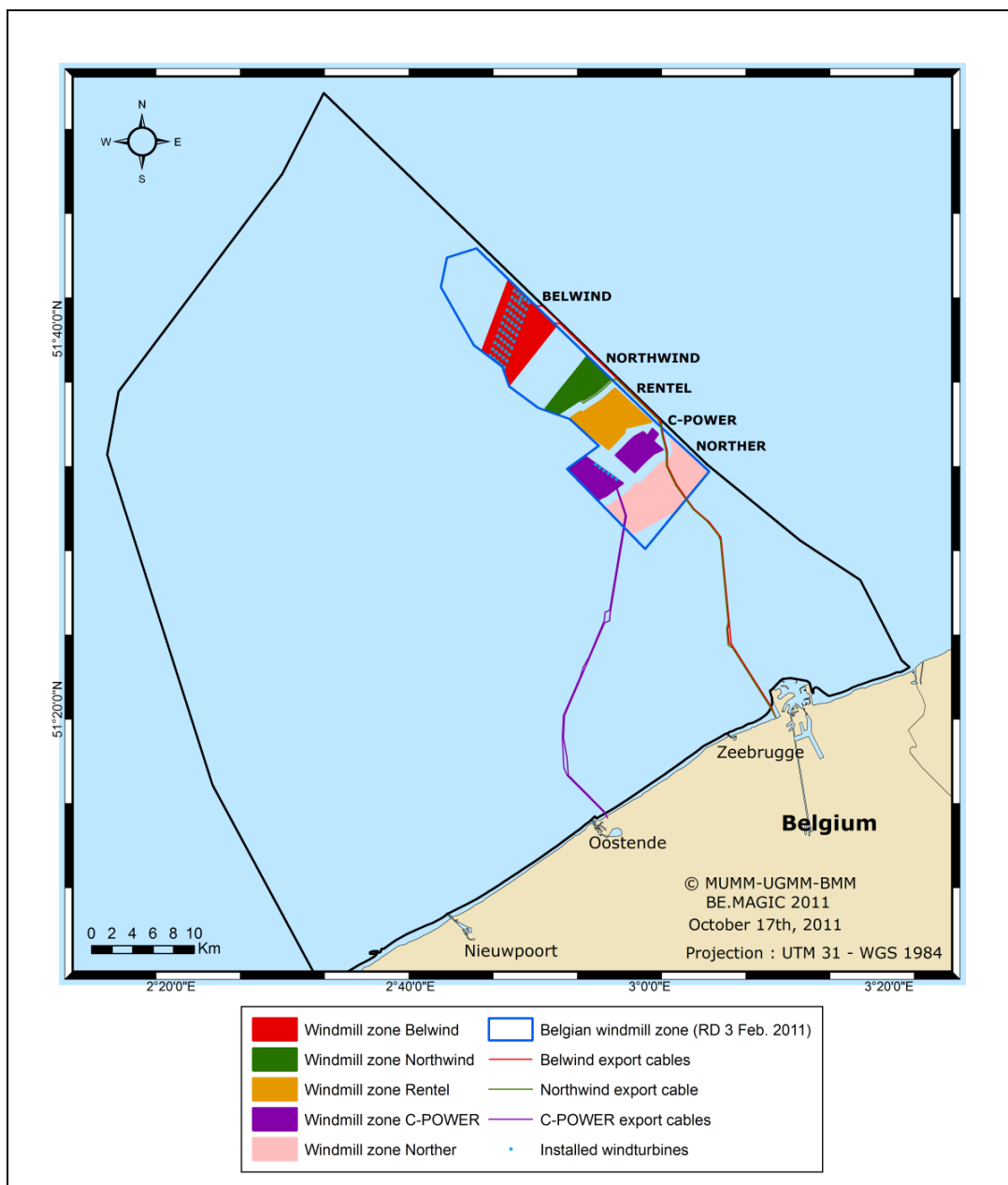
Afbeelding 7-1: Windturbinezones en kabels voor de uitvoer van elektriciteit
