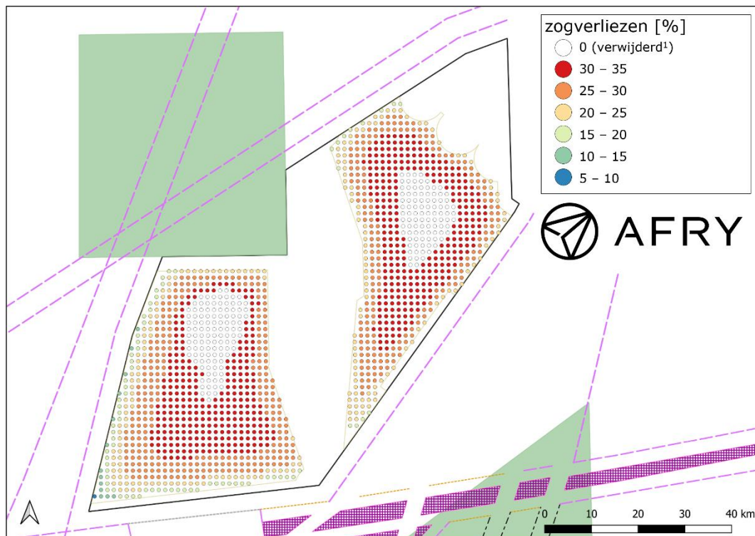
Figuur 21: #33 (Uiterste) turbinelayout met zogverliezen (Eddy Viscosity)
