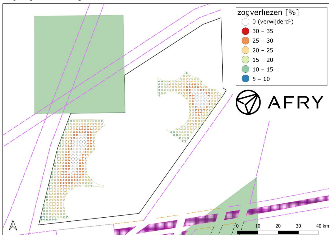
Figuur 20: #0 (Uiterste) turbinelayout met zogverliezen (Eddy Viscosity)
